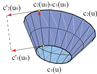
Figura 5: Superficie desarrollable
